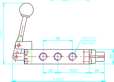
VBM 410-02 VBM 410-03
