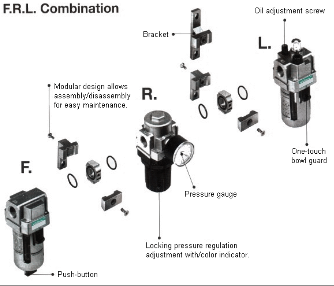
F.R.L.
